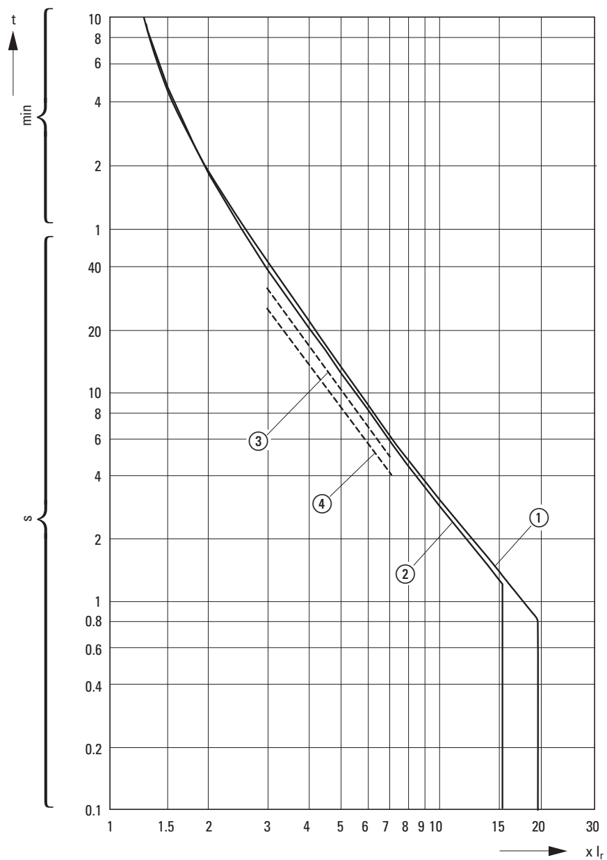
Abbildung/Figure 24: PKZM0-32/XTPR032BC1NL
