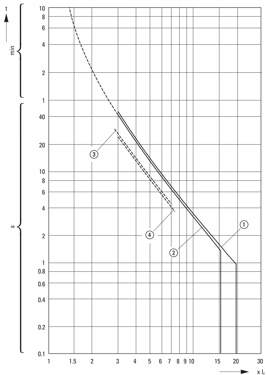
Abbildung/Figure 22: PKZM0-20/XTPR020BC1NL
