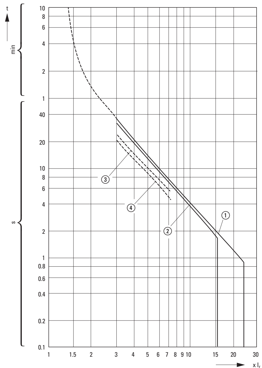
Abbildung/Figure 21: PKZM0-16/XTPR016BC1NL
