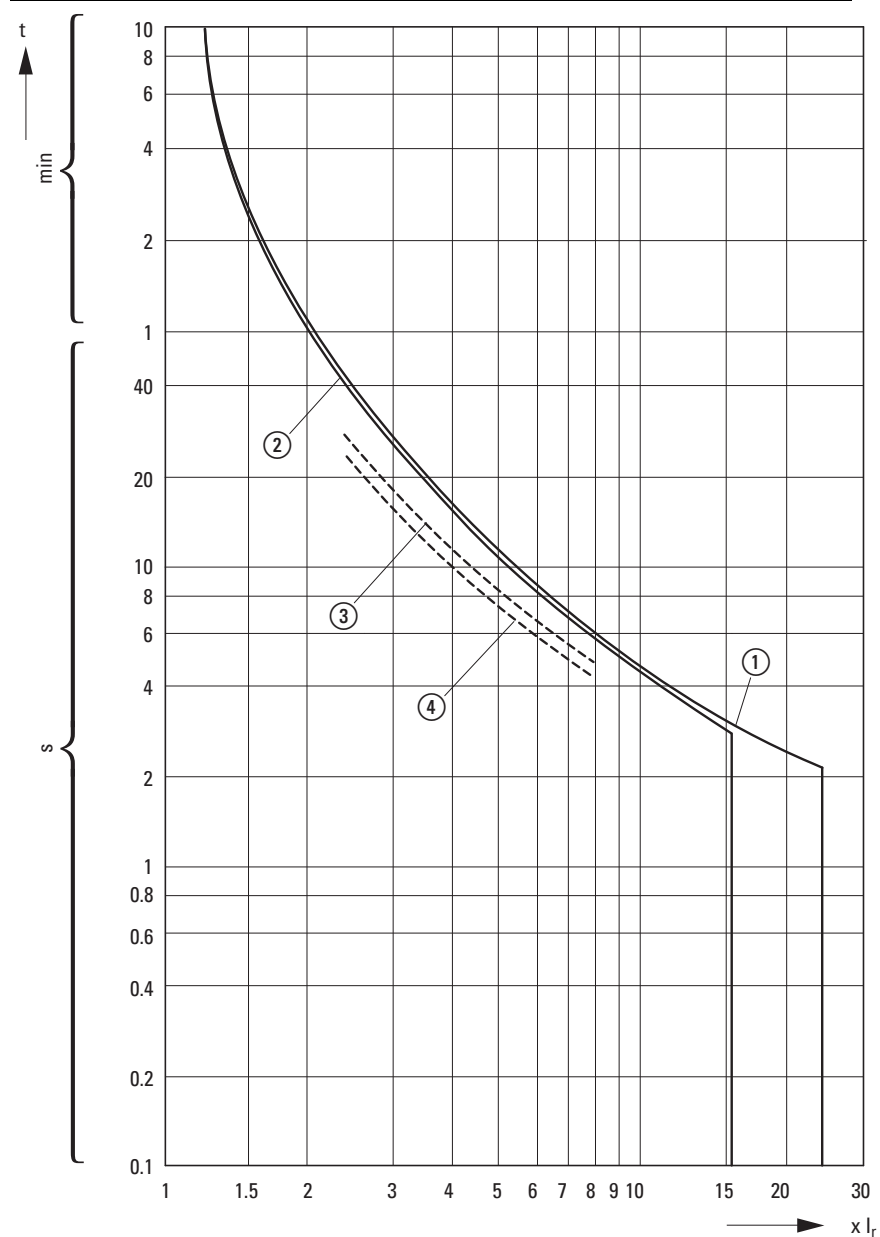
Abbildung/Figure 14: PZKM0-1/XTPR001BC1NL
