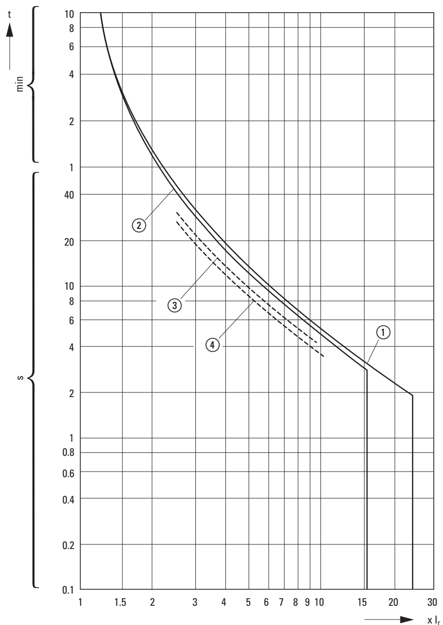
Abbildung/Figure 17: PKZM0-4/XTPR004BC1NL
